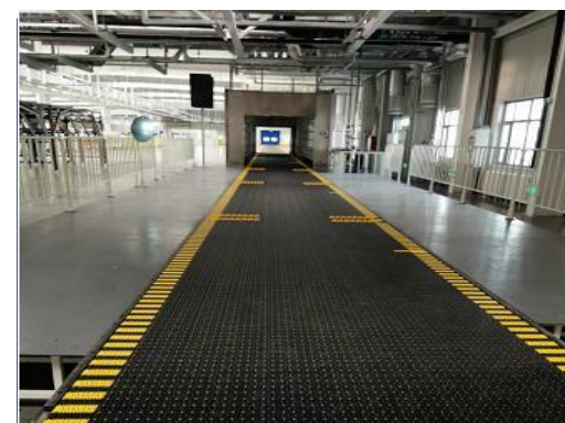
一汽丰田淋雨线 链网BM6992H8-K90 项目开始于2021年9月
